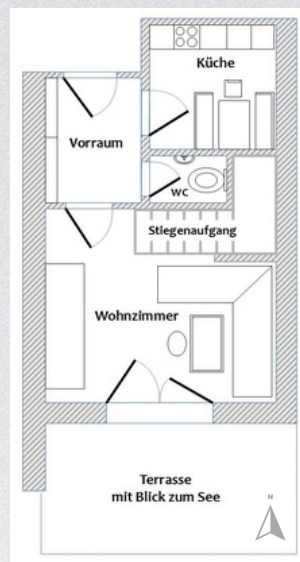
Erdgeschoss
